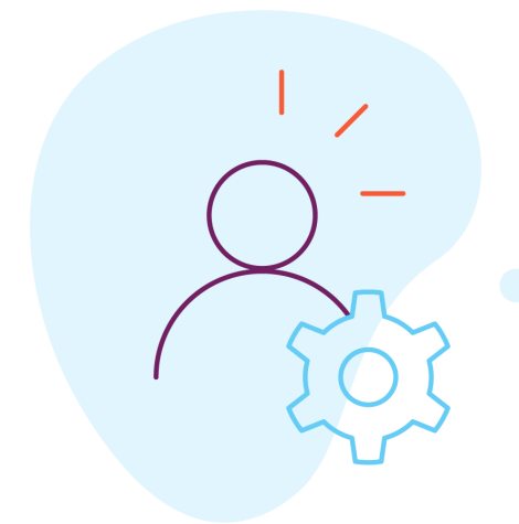
DevOps
